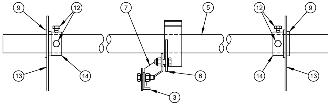
VIEW A-A
